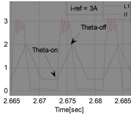
الشكل رقم (18): تيار الطور الأول مع محارضة الطور ذاته من أجل i_{ref} = 3A
