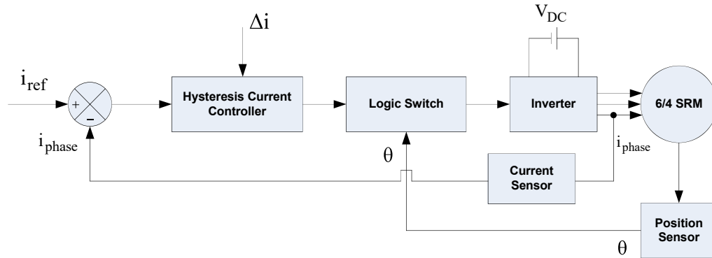
الشكل رقم (15): المخطط الصندوقي لقيادة المحرك SRM باستخدام نظرية التحكم بالتيار Hysteresis Controller
