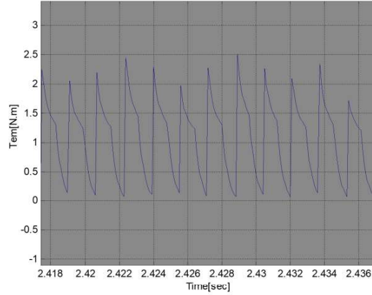
الشكل رقم (13): إشارة العزم اللحظي الكلي في المحرك SRM
