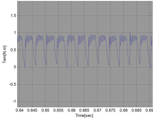
(a): إشارة العزم اللحظي للمحرك SRM
