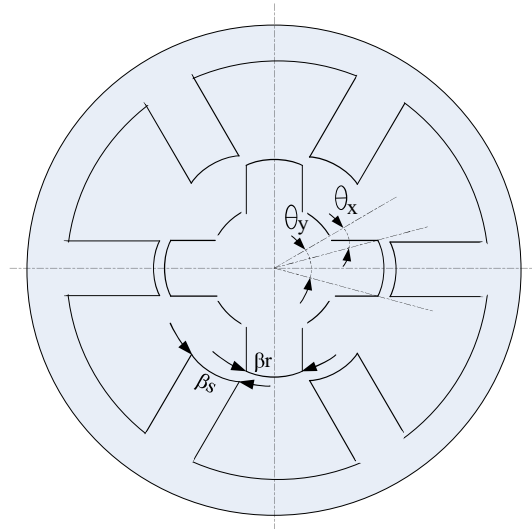
الشكل رقم (1): بنية المحرك SRM ذي النمط 6/4
