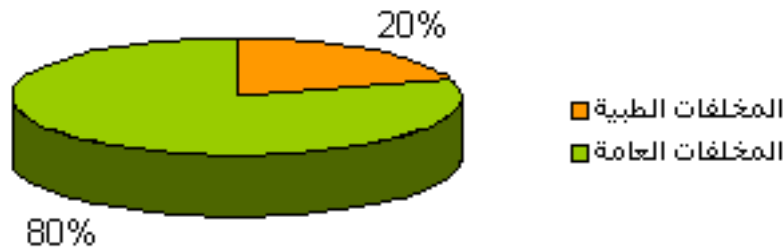
الشكل البياني رقم(١) نسب مكونات النفايات الطبية
