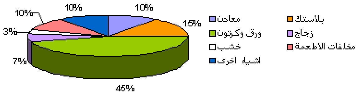
الشكل البياني رقم(٢) مكونات النفايات الطبية العامة
