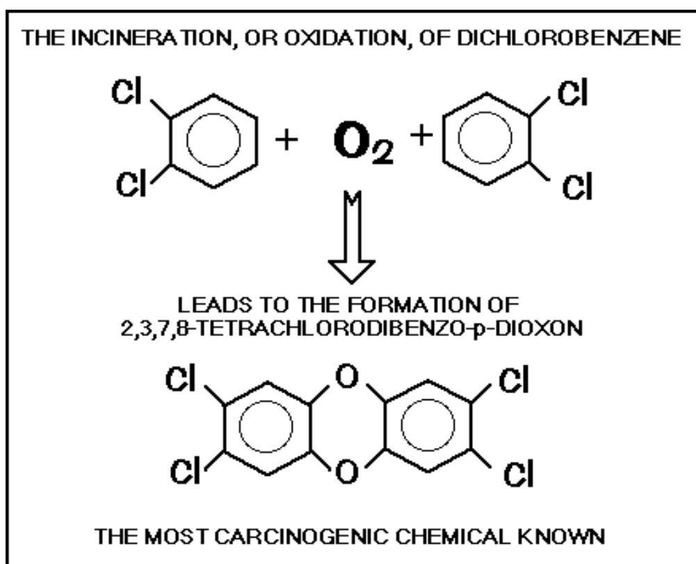
الشكل رقم (١) تشكل الديوكسين أثناء حرق النفايات الطبية
