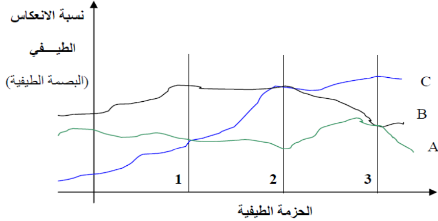
الشكل 1.8: البصمة الطيفية لثلاثة غطاءات أرضية
