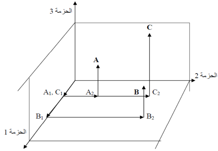
الشكل 2.8: تمثيل ثلاثي الأبعاد للنطاقات الطيفية الثلاثة
