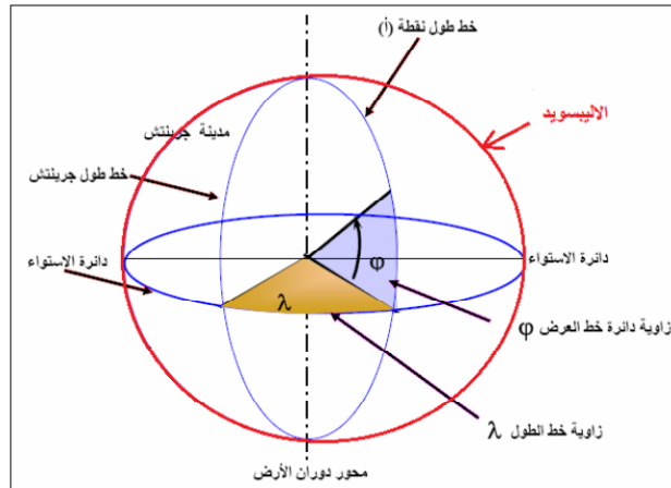
الإحداثيات الجيوديسية علي الألبيسويد
