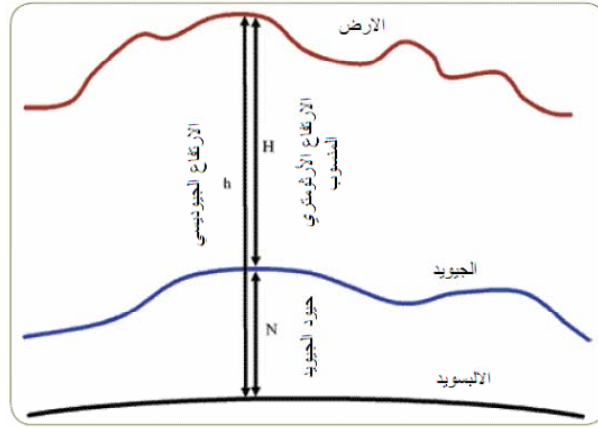
العلاقة بين الجيويد و الألبيسويد
