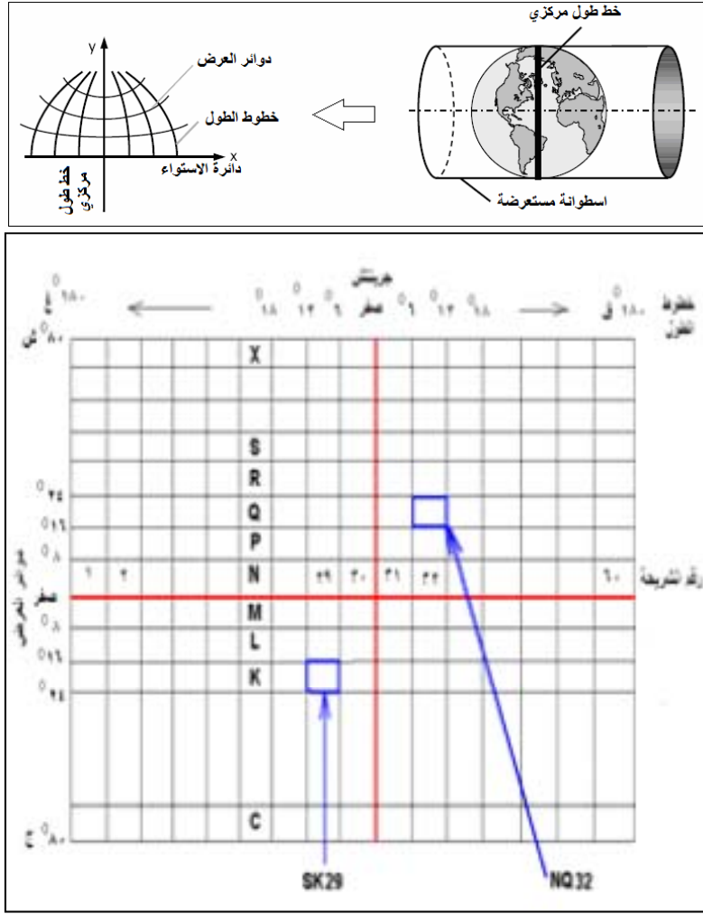
مسقط ميريكاتور المستعرض
