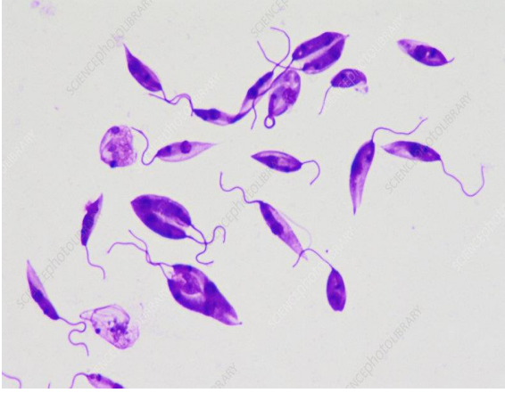
L. donovani
