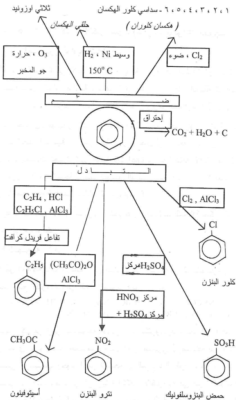
الشكل ( ٦ - ٣ ) مخطط تفاعلات البنزن
