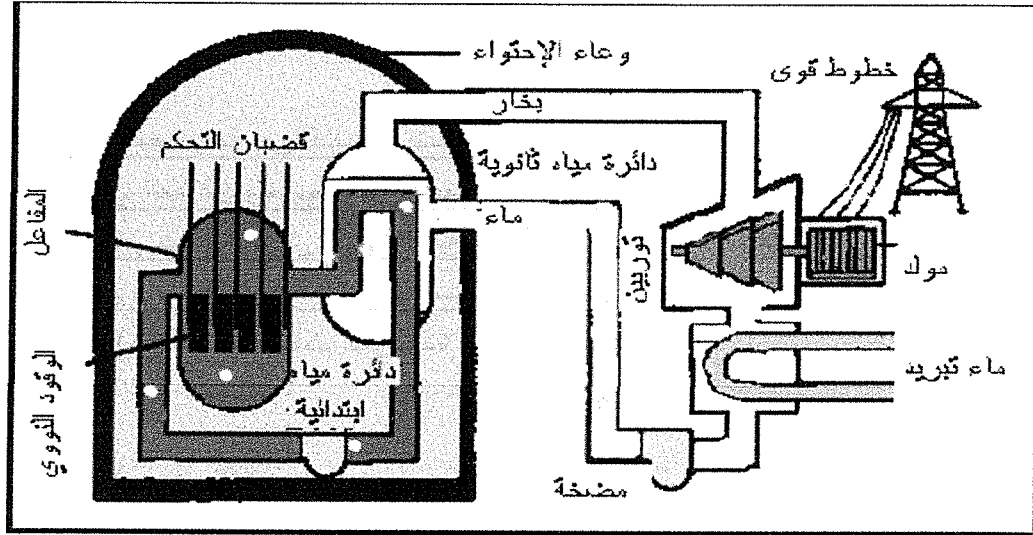
الشكل (٦) مفاعل نووي
