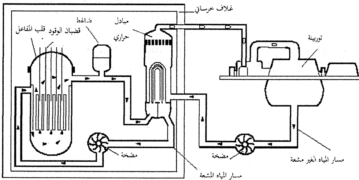
الشكل (٥) رسم تخطيطي لمفاعل نووي
