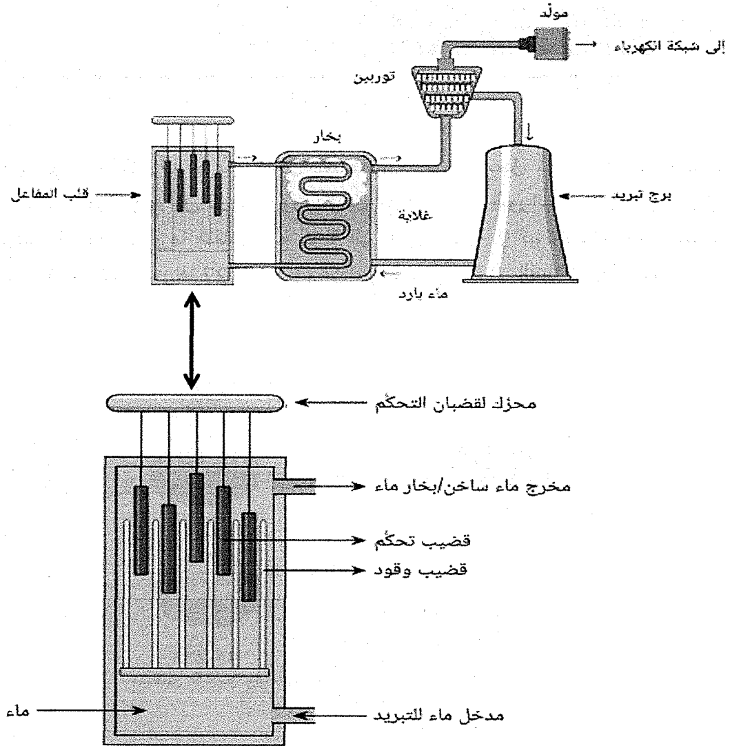
الشكل (٨) قضبان التحكم داخل قلب المفاعل
