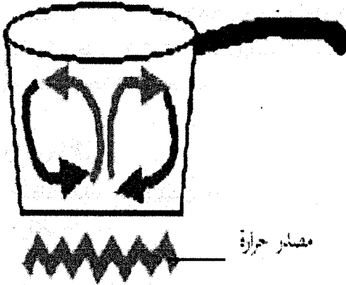
الشكل (١٠) رسم توضيحي لانتقال الحرارة بالحمل
