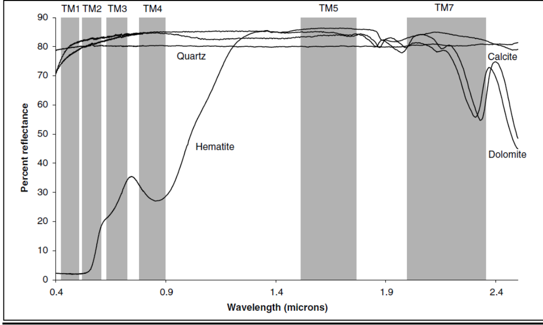
نسبة الأشعة المنعكسة من بعض المعادن لكل طول موجي
