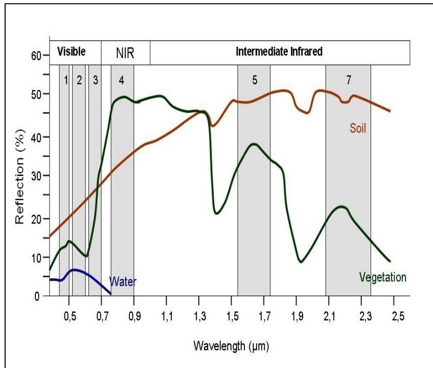
نسبة الأشعة المنعكسة من التربة و النبات و الماء لكل طول موجي
