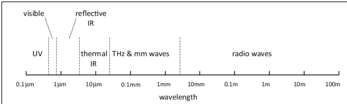
المجال الكهرومغناطيسي
