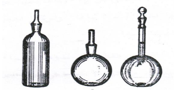
الشكل رقم (٤-٢): يوضح أشكال مختلفة من البكنوميترات لقياس الكثافة الحقيقية
