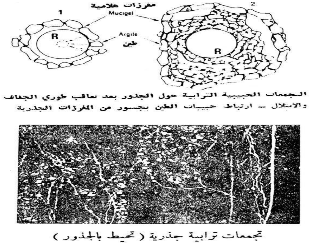
الشكل رقم (4): آلية تشكل التجمعات الترابية الجذرية
