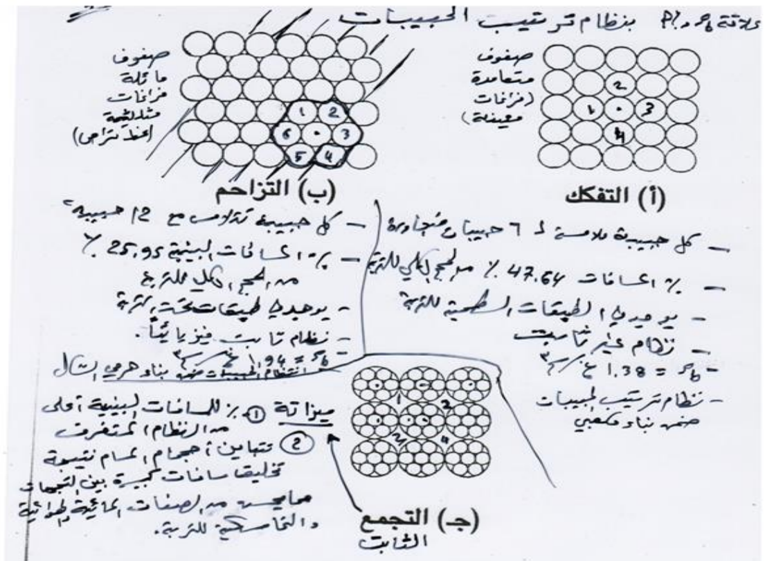
الشكل رقم (1) يبين تأثير نظام ترتيب الحبيبات في بعض الخصائص الفيزيائية للترربة
